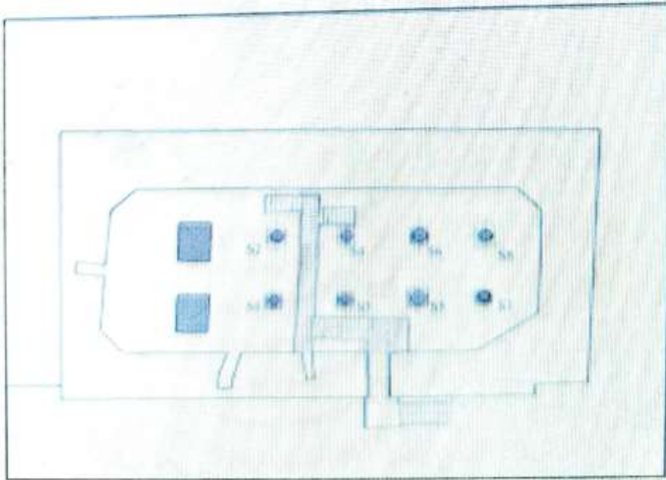
Şekil 3. 30 Askeri Depolar Komutanlığı sarnıcı planı (IRAM Arşivi, çiz: Ayşenur Çucenoğlu, 2013)
